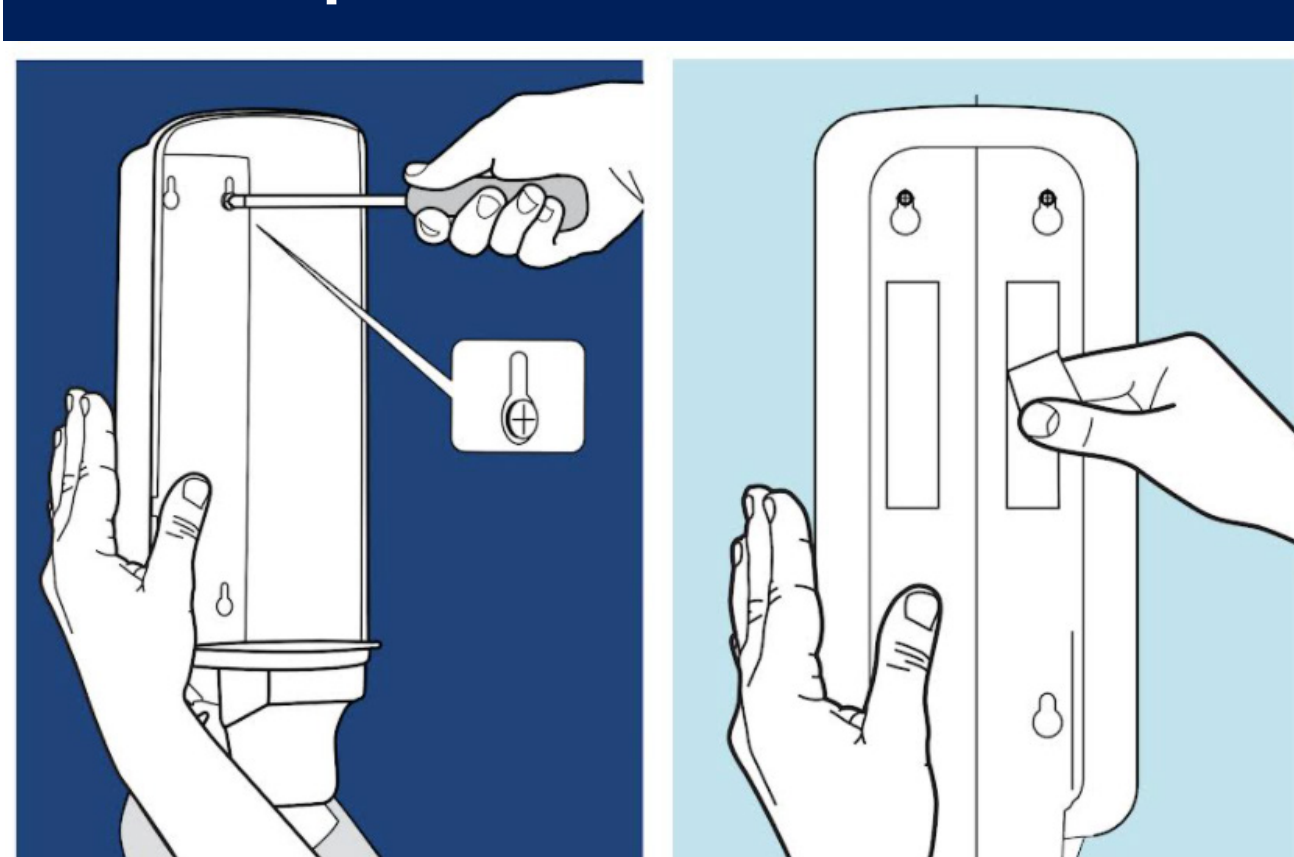
Montaje con tornillos
